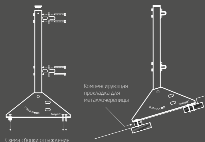
Схема сборки ограждения
