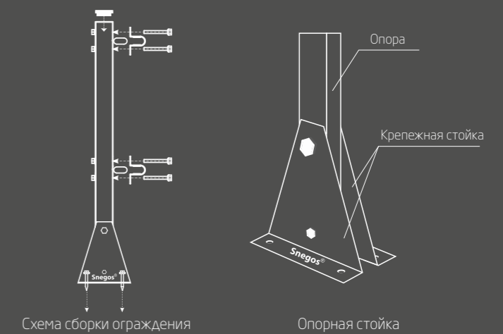
Схема сборки ограждения
