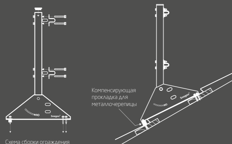
Схема сборки ограждения
